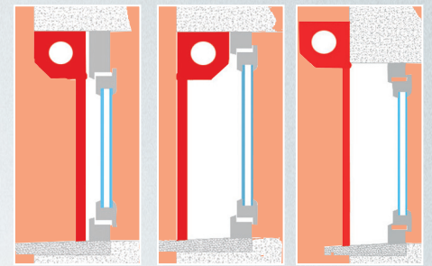
Pose enroulement extérieur Pose enroulement intérieur Pose en applique ou en façade
